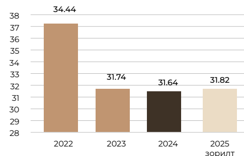
Нэгж бүтээгдэхүүнд ногдох эрчим хүч /кВт.ц/ш/*
