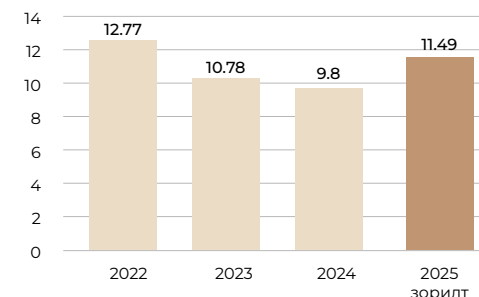
Нэгж бүтээгдэхүүн үйлдвэрлэлээс ялгарах хүлэмжийн хий /кгCO2/
